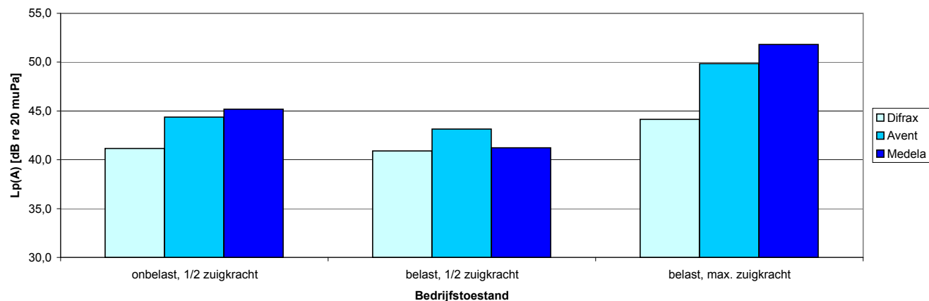
Geluiddrukniveau Lp(A) (indicatief) voor een gebruiker in een woonkamer
