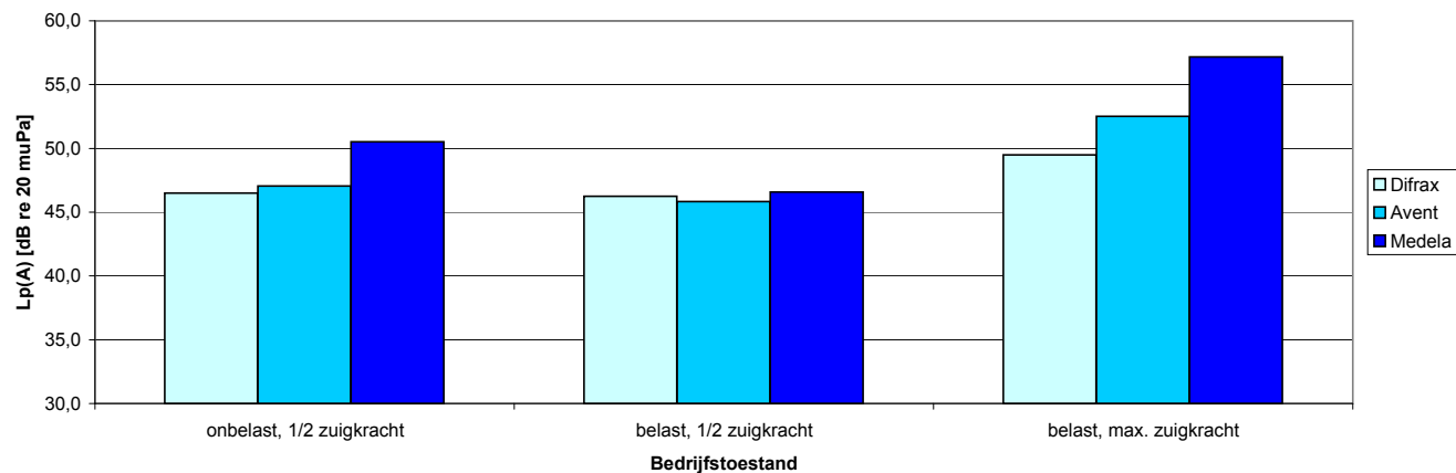
Geluidvermogen Lw(A) (exact)
